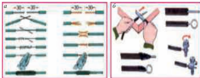
Расми 22. Таъмири ноқили кандашуда. Ҳалқакунӣ ва пайвасткунии пайдарҳами симҳо.
