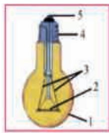
Расми 23. Сохти лампочкаи рӯзгор: 1 - шиша; 2- мӯяки тафсанда; 3- электродҳо; 4- печтоб; 5- ит-тисоли марказӣ.
